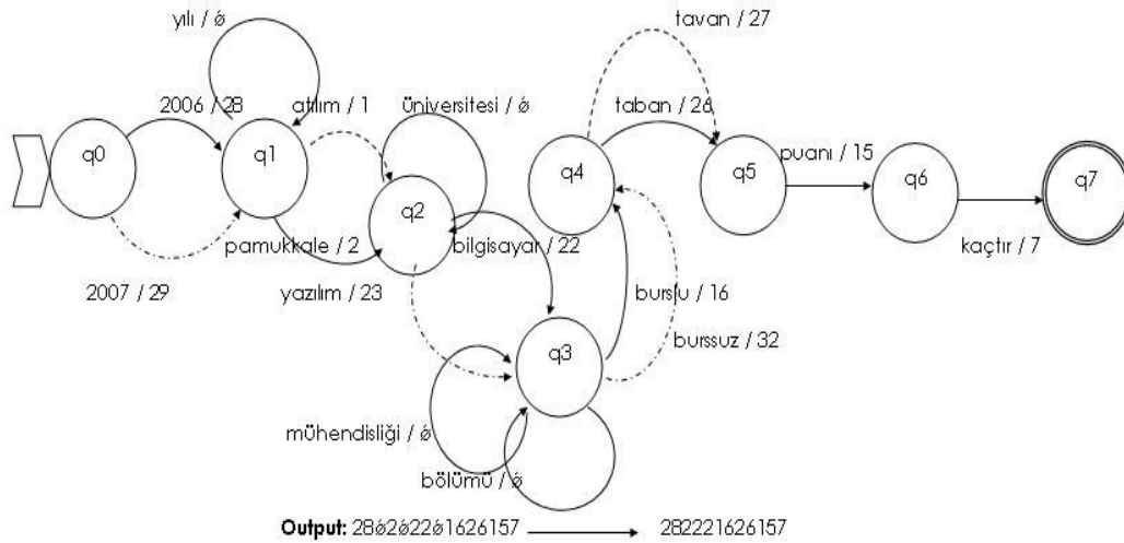
Figure 4.4 Mealy machine for the question “2006 yılında pamukkale üniversitesi bilgisayar mühendisliği bölümü burslu taban puanı kaçtır?”
