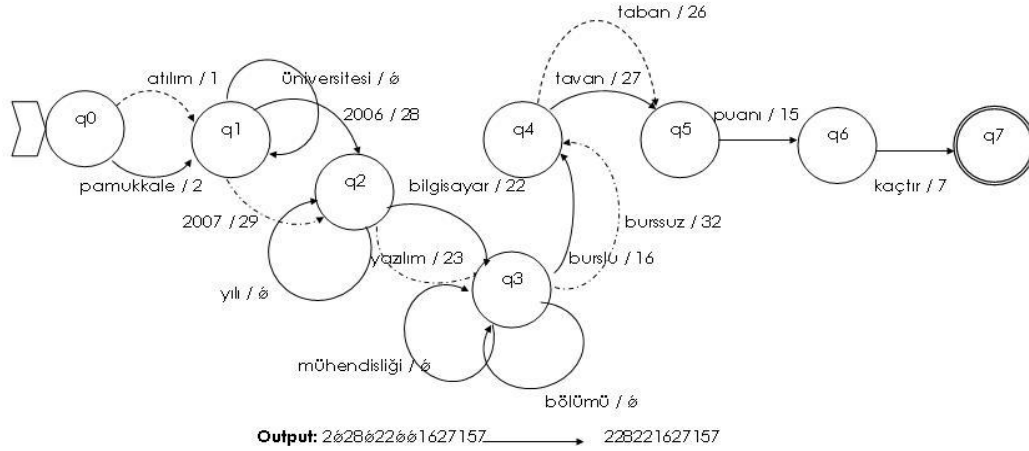
Figure 4.5 Mealy machine for the question “pamukkale üniversitesi 2006 yılındaki bilgisayar mühendisliği burslu tavan puan kaçtır?”
