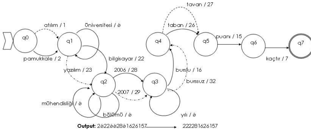
Figure 4.3 Mealy machine for the question “Pamukkale üniversitesi bilgisayar mühendisliği bölümünün 2006 yılı burslu taban puanı kaçtır?”
