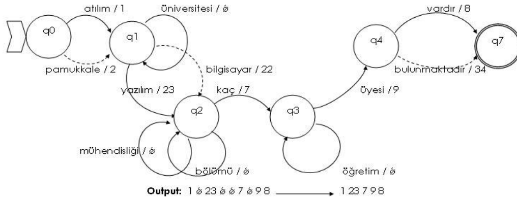
Figure 4.2 Mealy machine for the question “Atılım üniversitesi yazılım mühendisliği bölümünde kaç öğretim üyesi vardır?”
