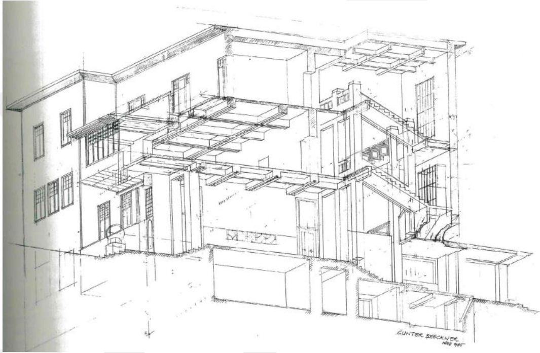
Şekil 5.90 Merkezi Eksen Boyunca Aksonometrik Kesit, 1985 (Breckner, 1985'ten akt. Kapfinger, 2021, 11)
