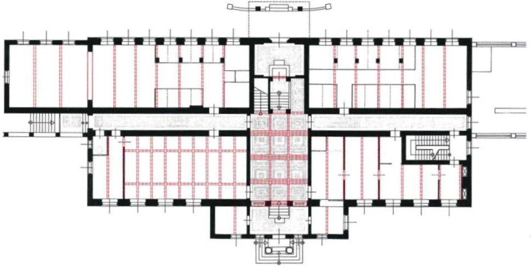
Şekil 5.82 Yükseltiilmiş Zemin Kat Planı, 1982 (Tavandaki Kirişler Kırmızı Renk ile Gösterilmiştir, Eklemeler Manuel Kainz, 2020) (Kapfinger, 2021, 113)
