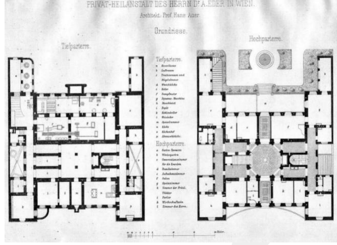
Şekil 5.4 Fürth Sanatoryumu Bodrum Kat ve Yükseltilmiş Zemin Kat Planı (Auer, 1888, Bl.4)
