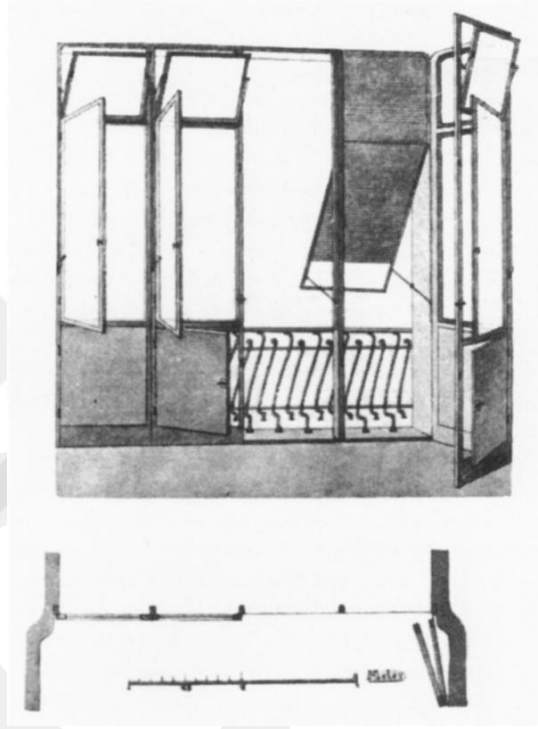
Şekil 5.73 Hareketli Cam Paneller, Dr. Karl Turban, 1902 (Topp, 1997, 421)
